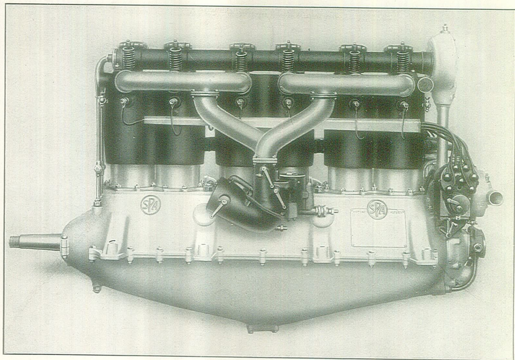
• Motore 6 A Surcompresso - Lato carburatore.
